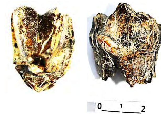
Рис. 2. Верхний коренной зуб Gobiatherium mirificum : а – вид с жевательной поверхности, б – сбоку
