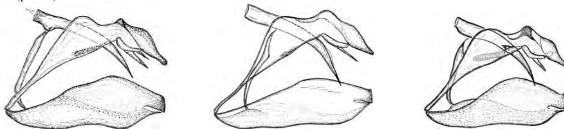
Рис. 1-3. Строение гениталий самцов рода Plebejus (вид сбоку): 1 – Pl. sarydzhazi , sp. n. (paratypus); 2 – Pl. arina (paratypus); 3 – Pl. idas (topotypus)
