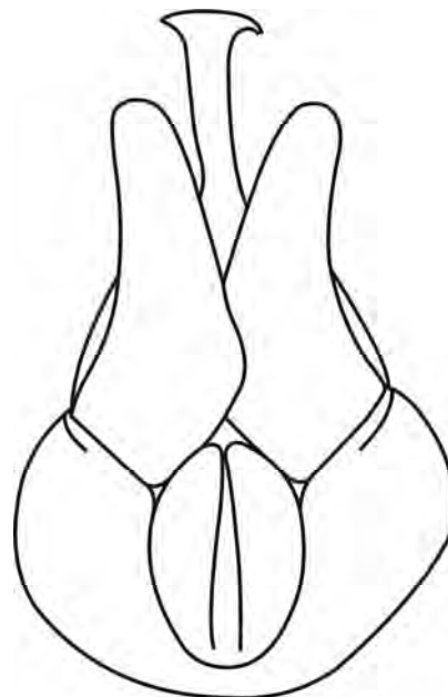
Рис. Гипопигий Chrysotoxum bicinctum bakhtjarovi ssp. n. Вид снизу.
