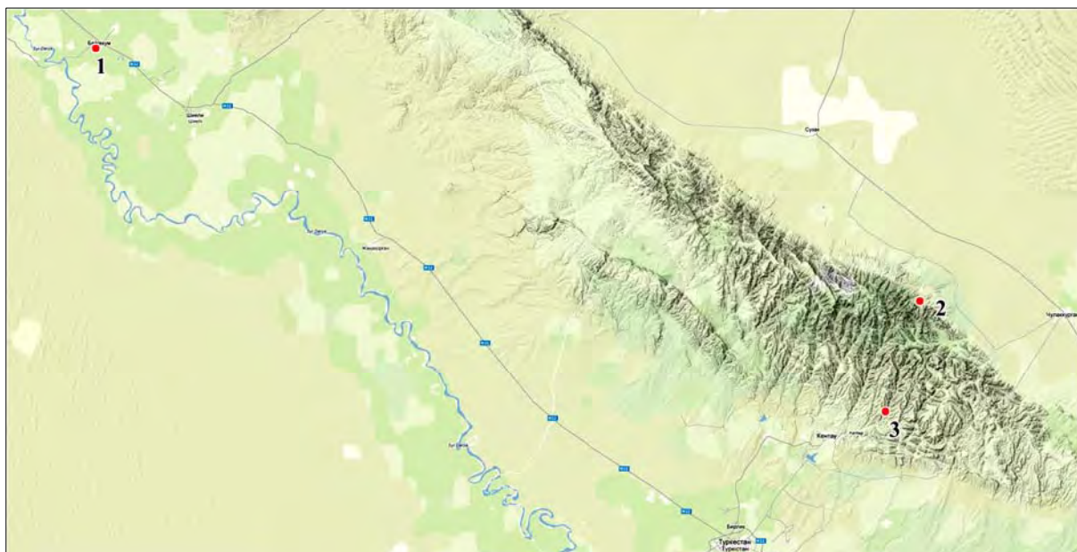
Рис. 4. Распространение M. glasnovi .
