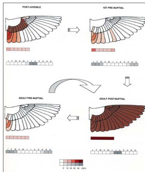
Рис. 3. Схема линьки пустынной славки (Schirihai et al., 2001)
